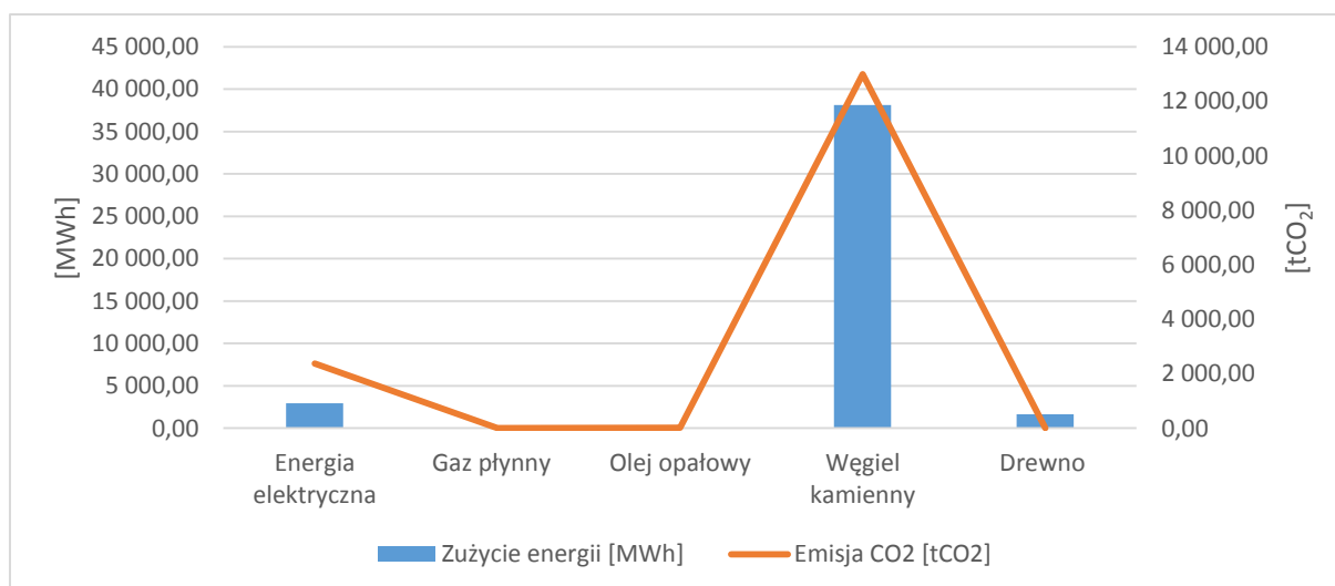
Rysunek nr 18. Łączne zużycie poszczególnych nośników energii wraz z produkcją CO 2 w budynkach mieszkalnych
