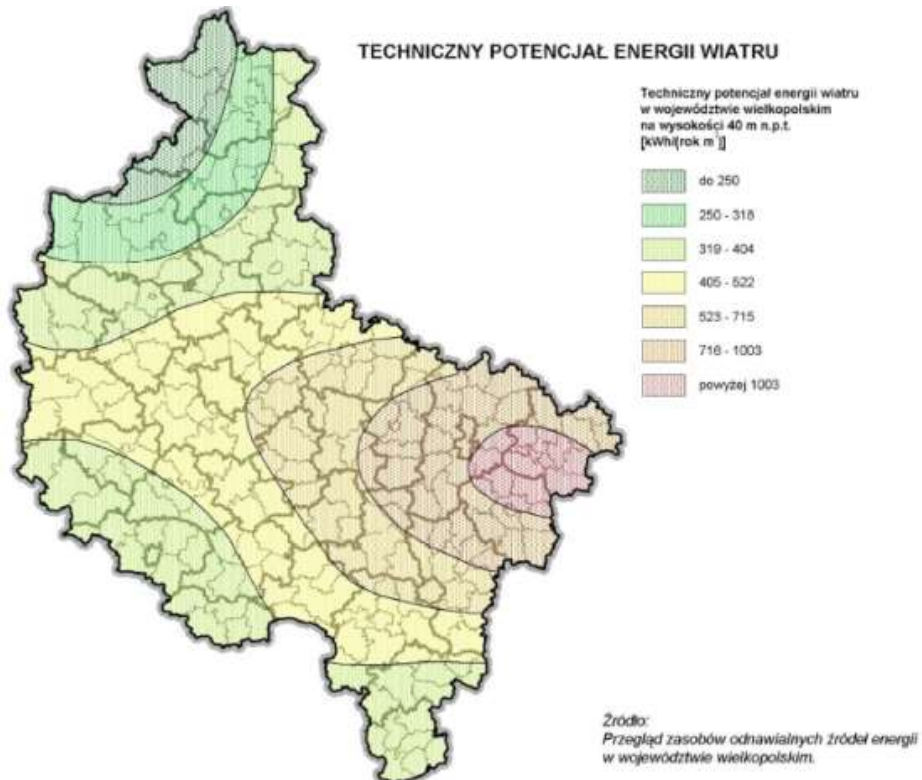
Rysunek nr 10. Techniczny potencjał energii wiatru dla Wielkopolski i poszczególnych powiatów
