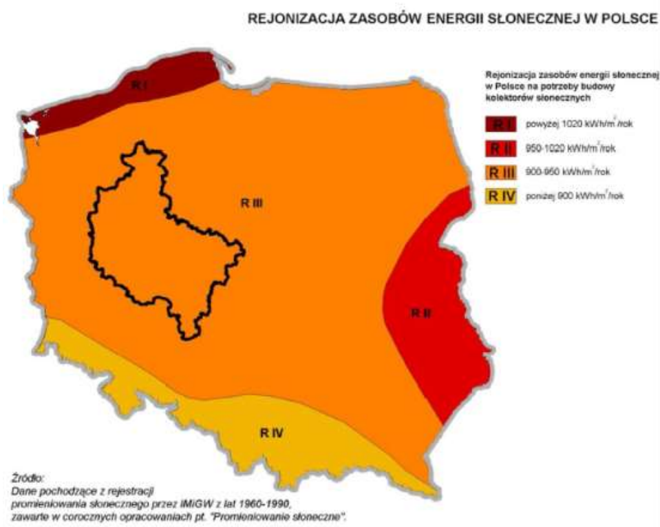
Rysunek nr 11. Rejonizacja zasobów energii słonecznej w Polsce Źródło: Energetyka odnawialna w Wielkopolsce uwarunkowania rozwoju, Poznań 2012
