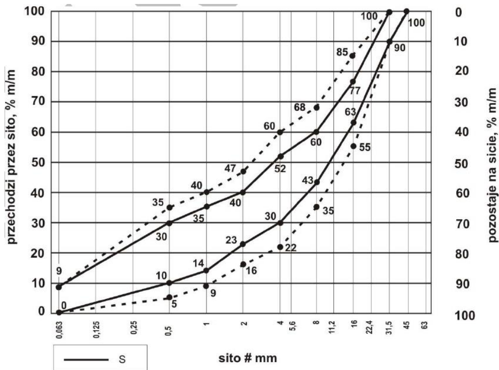
Rysunek nr 2. Mieszanka kruszyw 0/31,5 do warstw podbudowy pomocniczej (mieszanka niezwiązana wg WT-4)
